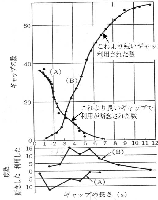
図 2-27 合流車が本線走行車のギャップを利用した数と断念した数(【交通工学 HB2001】4.6.2 節, 図 4.6.14)
