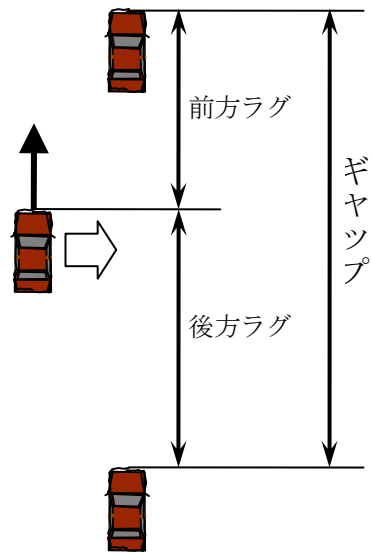
図 2-28 ギャップと前方ラグと後方ラグ
