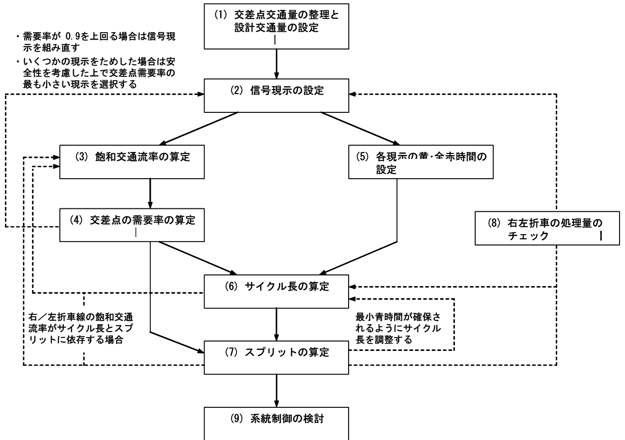
図 5-9 信号表示案の設計手順 (【交通信号手引】3 章参照)
