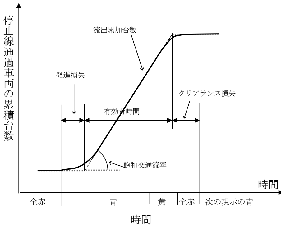
図 5-7 1つの現示における損失時間
