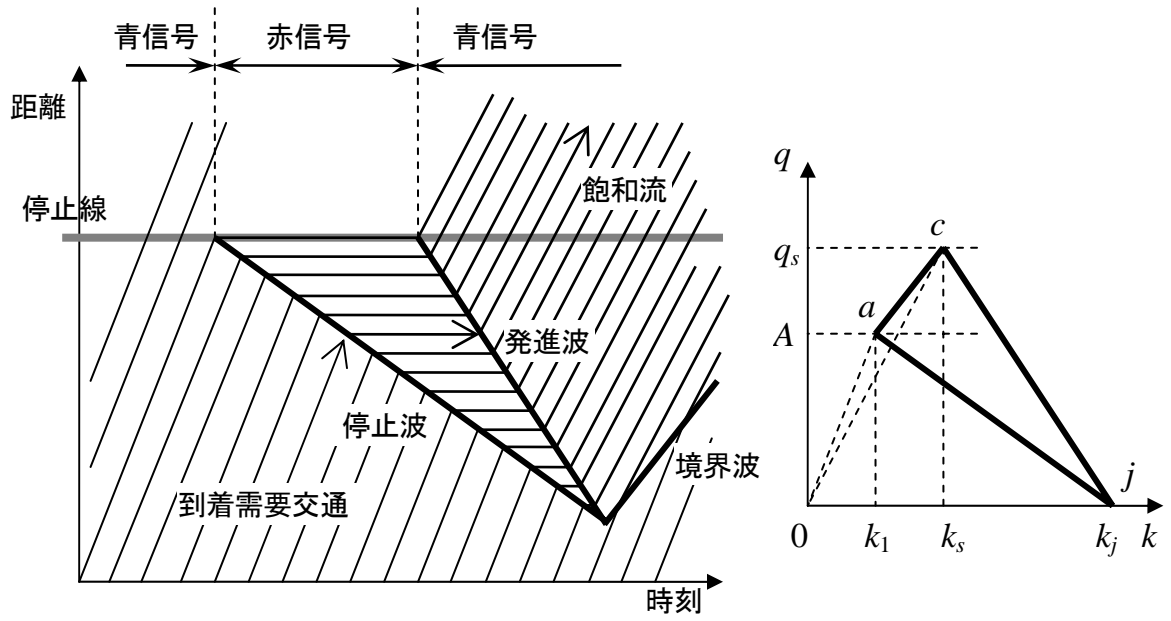
図 2-26 時間・距離図上の停止波・発進波と q-k 図との関係
