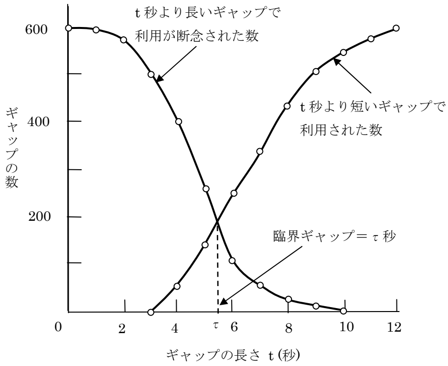
図2-25 ギャップアクセプタンス挙動
